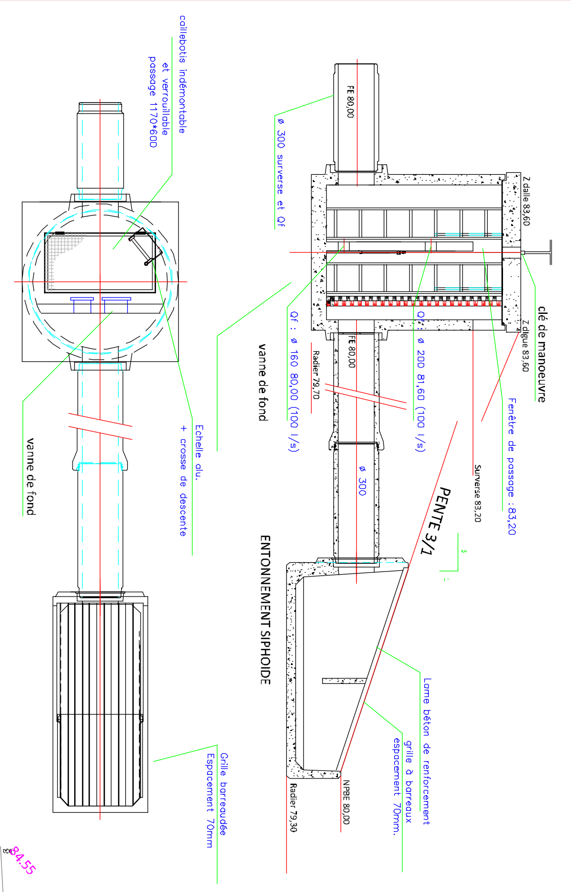
Profil de l'ouvrage de fuite - Barrage enherbé
